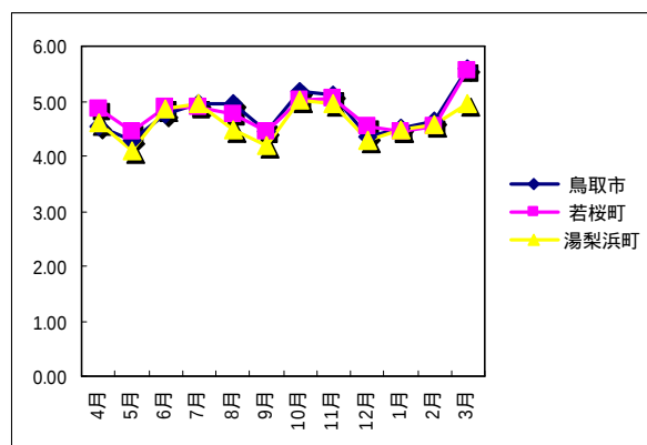
図 1 平成 21 年度における pH の経月変化
