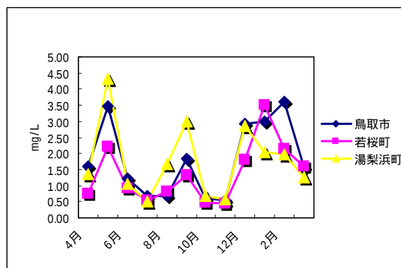
図 3 平成 21 年度における \text{NO}_3^- 濃度の経月変化
