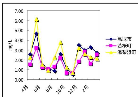
図 2 平成 21 年度における \text{nss-SO}_4^{2-} 濃度の経月変化
