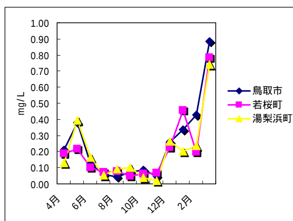
図 4 平成 21 年度における \text{nss-Ca}^{2+} 濃度の経月変化
