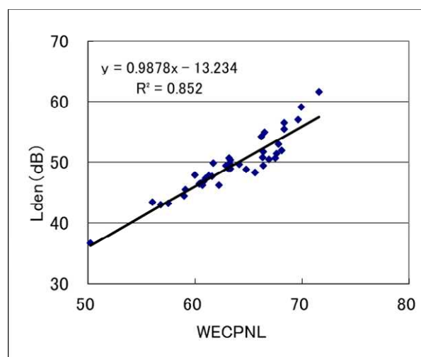
図4 Lden と WECPNL との相関(N=42)
